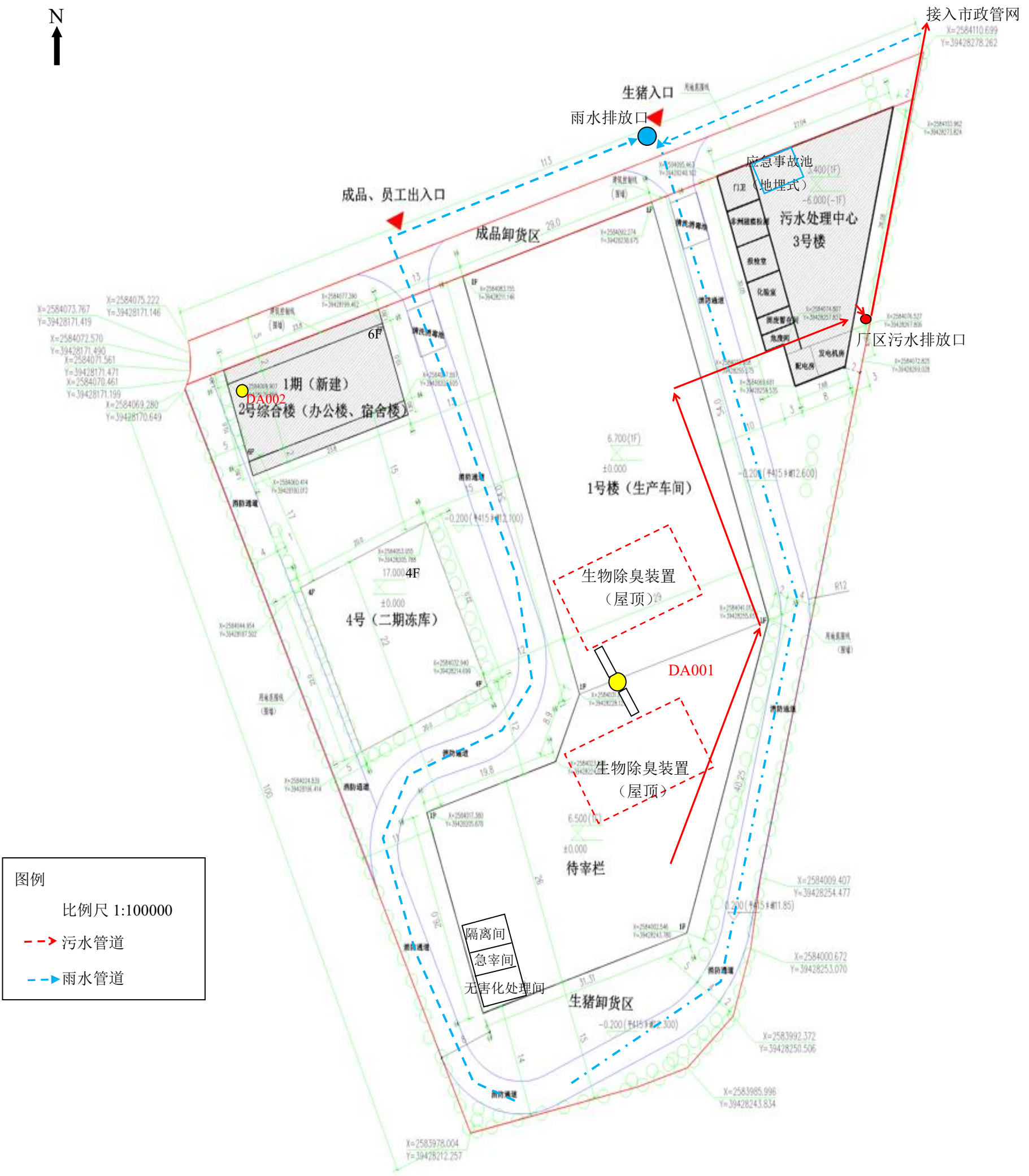
图 3.1-1 原环评项目厂区总平面布置图
