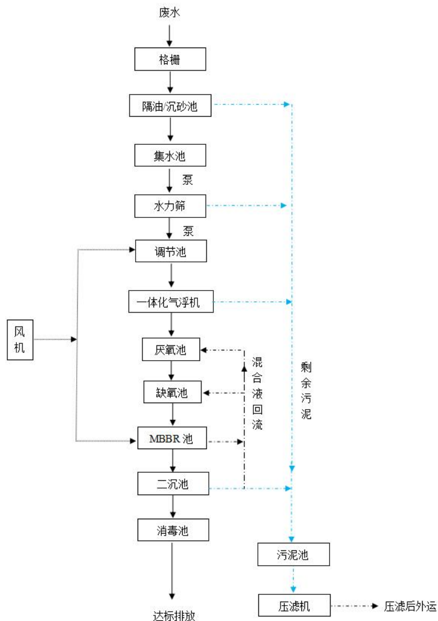
图 8.1-1 综合废水处理工艺流程图
