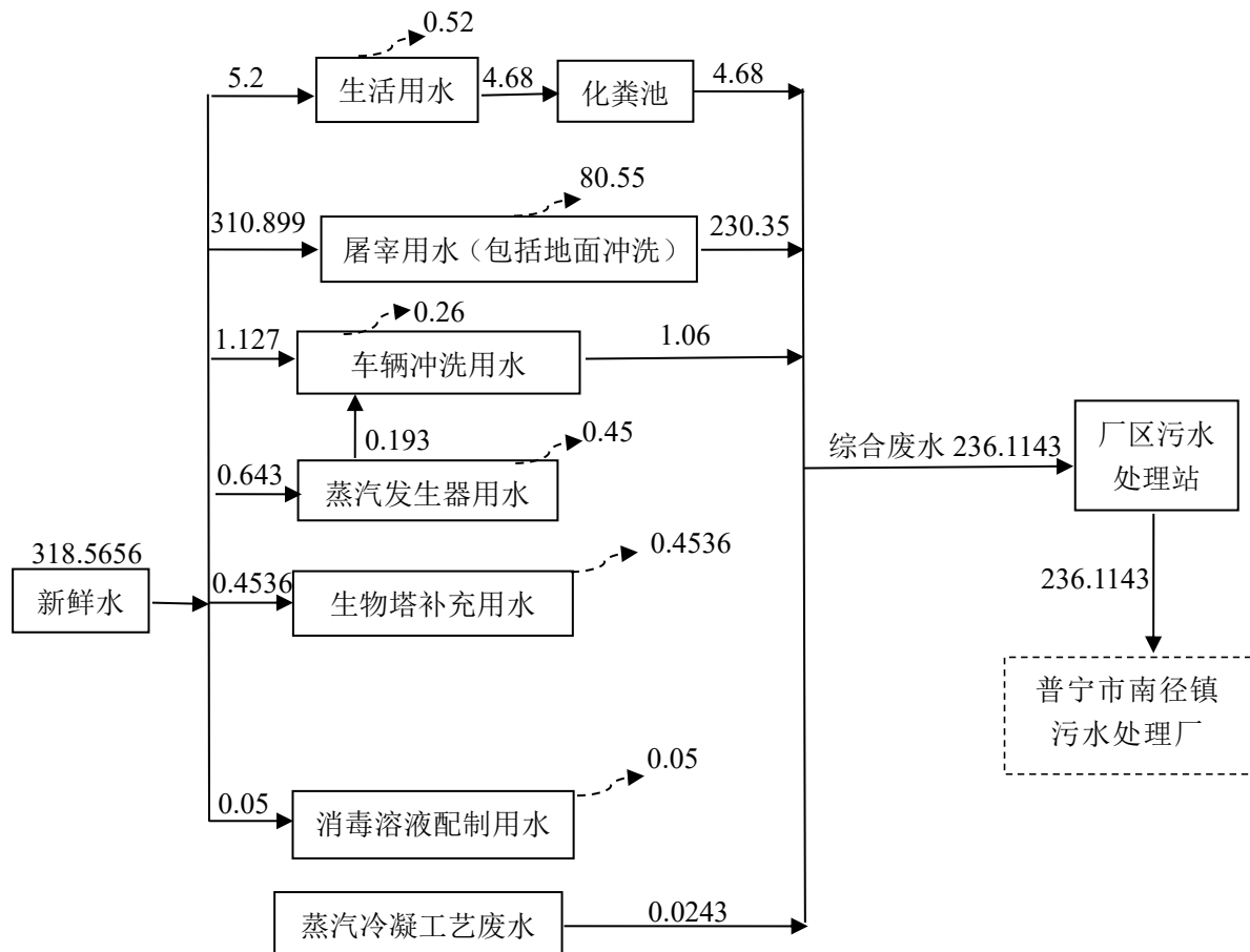
图 4.4.2-1 本项目水平衡图（单位：t/d）
