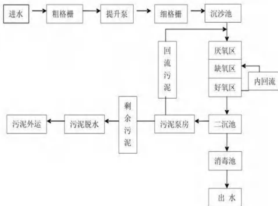
图4.2-1 揭阳市榕城区仙梅污水处理厂工艺流程图
