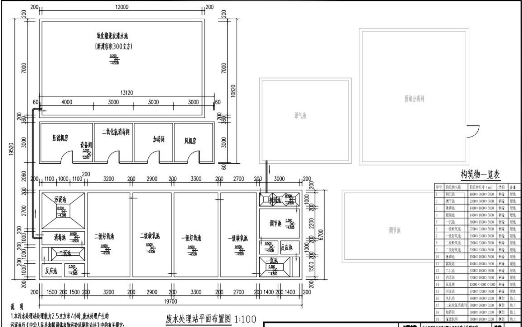
图 2-11 污水站平面布置图
