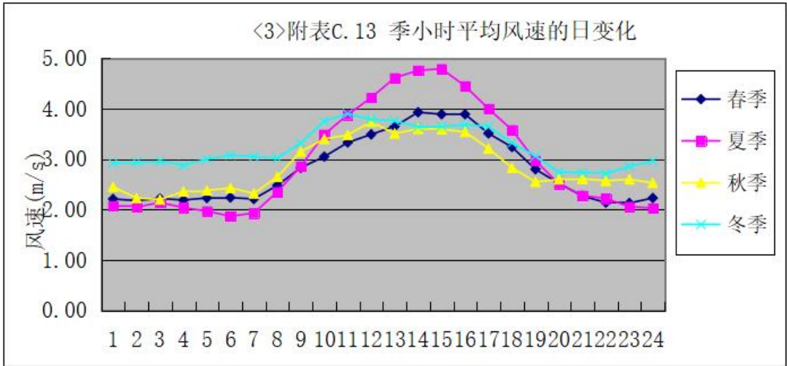
图 4.2-4 各季小时月平均风速变化曲线
