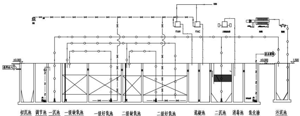
图 5.2-1 建设项目污水处理系统工艺流程图示
