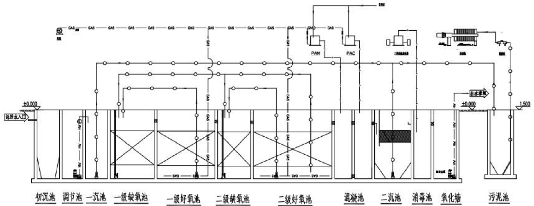
图 2-13 污水设施工艺流程
