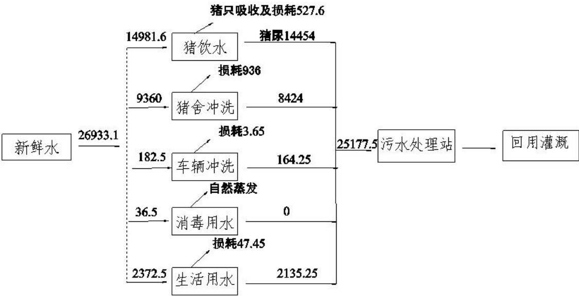
图 2-14 扩建后全厂水平衡图 (单位: t/a)
